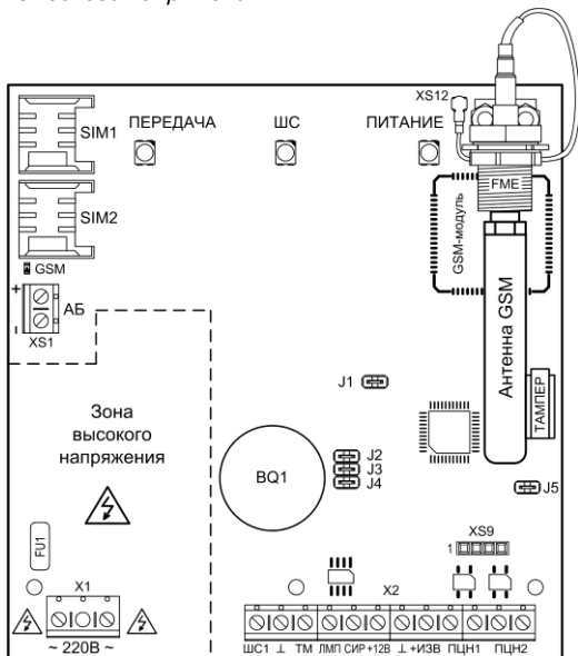
Рис.1 Плата прибора
