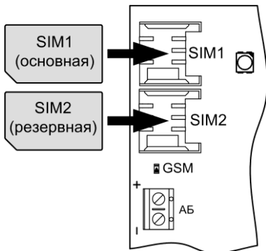
Рис.6 Установка SIM-карт
